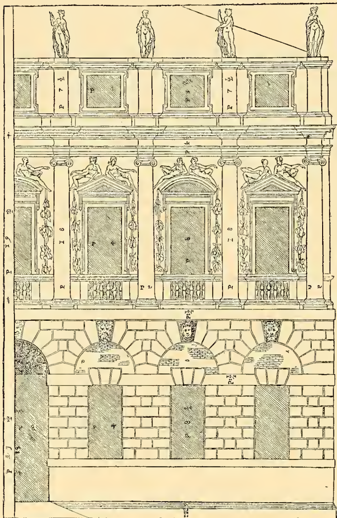
Projet de palais, par Palladio. (Traité d'architecture, liv. II.)
